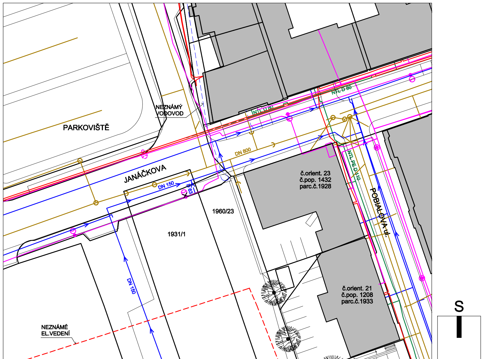
SITUACE M 1:500 BYTOVÝ DŮM JANÁČKOVA-MASNÁ, MORAVSKÁ OSTRAVA
